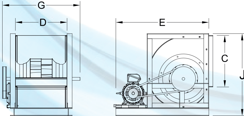
CENTRIFUGAL FAN ( BACKWARD CURVED)-DIDW
